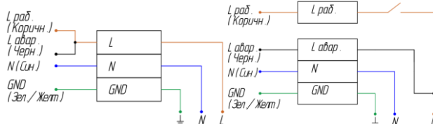
а) без выключателя (постоянный режим); б) с выключателем (включение/выключение рабочего освещения).
